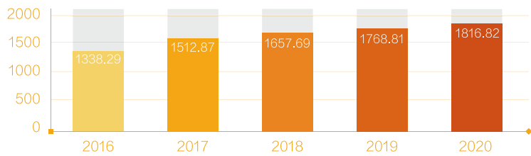
“十三五”期间山西省内售电量（亿千瓦时）
