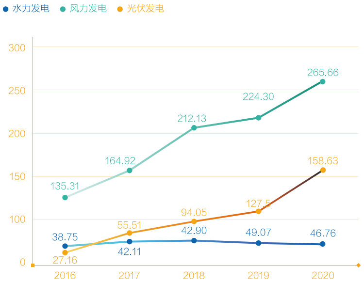
“十三五”期间水力发电、风力发电、光伏发电发电量（亿千瓦时）
