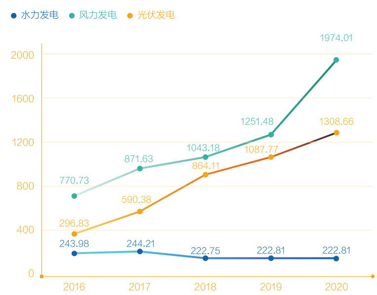
“十三五”期间水力发电、风力发电、光伏发电并网容量（万千瓦）
