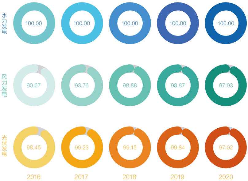
“十三五”期间水力发电、风力发电、光伏发电利用率（%）
